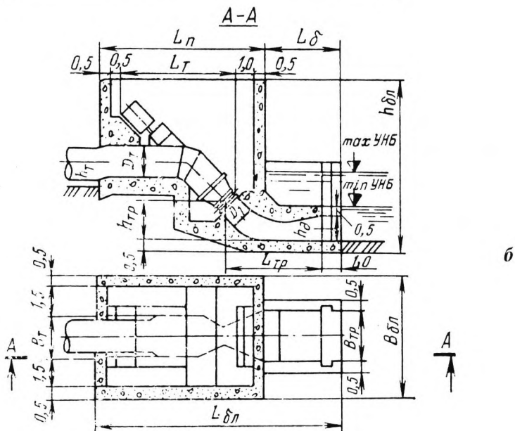
Рис.5.8. Здание ГЭС кожуховым подводом воды а-с горизонтальной осевой турбиной; б- с наклонной турбиной
