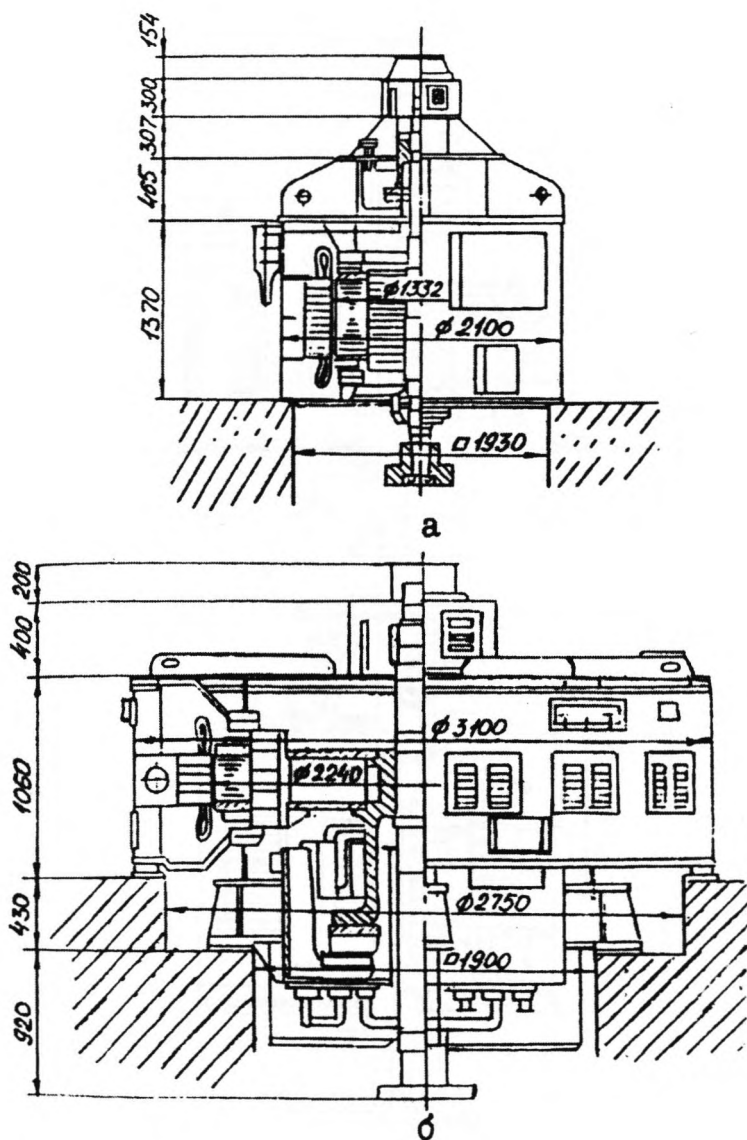
Рис. 2.14. Гидрогенераторы СВ173/56-14УХЛ4 (а) и СВ260/26-20УХЛ4 (б)
