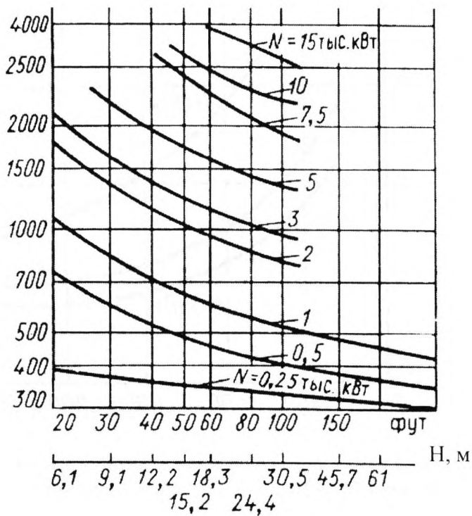
Рис.4.1. Стоимость строительства малых ГЭС в США
