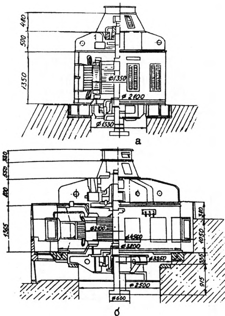
Рис. 2.15. Гидрогенераторы СТ173/59-10УХЛ4 (а) и СВ260/49-16УХЛ4 (б)
