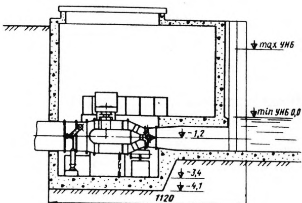
Рис.5.20. Компоновка здания малой ГЭС с горизонтальной капсульной гидротурбиной и вынесенным в машинный зал вертикальным генератором
