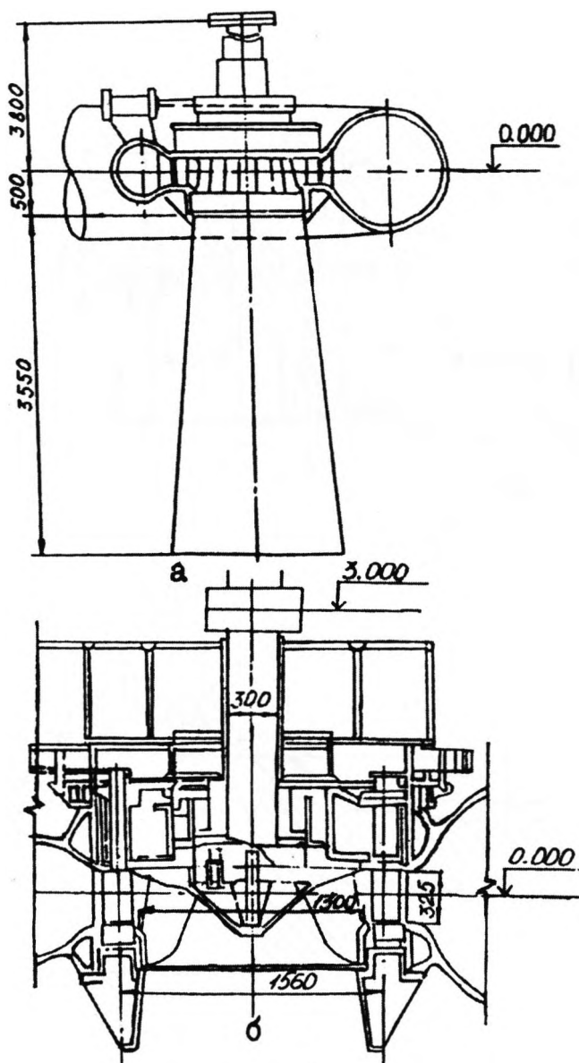
Рис. 2.9. Гидротурбины P0140/871-B-112 (а) и P0170/803-B-130 (б)
