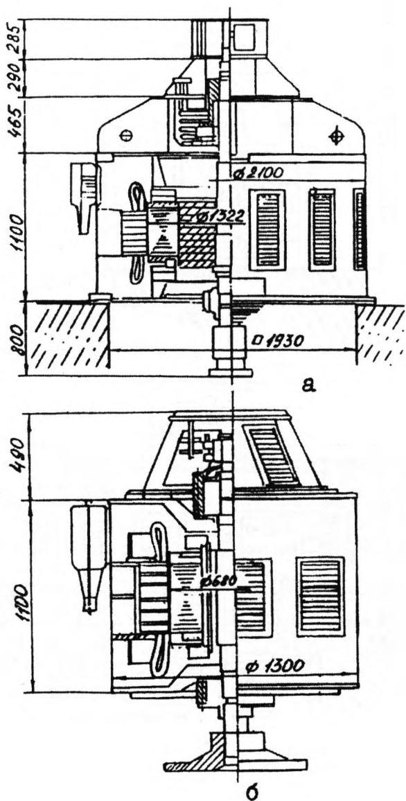
Рис. 2.13. Гидрогенераторы СВ173/28-14УХЛ4 (а) и СВ99/41-6УХЛ4 (б) 27
