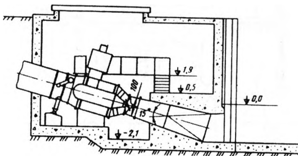
Рис.5.18. Компоновка здания малой ГЭС при наклонном положении капсульной гидротурбины
