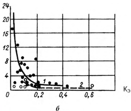
Рис.1.2. Графики зависимости K_{Э}=f(\frac{Э}{L}) а - реки Сибири и Дальнего Востока; б - реки Средней Азии и Казахстана; 1- реки мощностью 100000-200000 кВт; 2- реки мощностью свыше 200000 кВт
