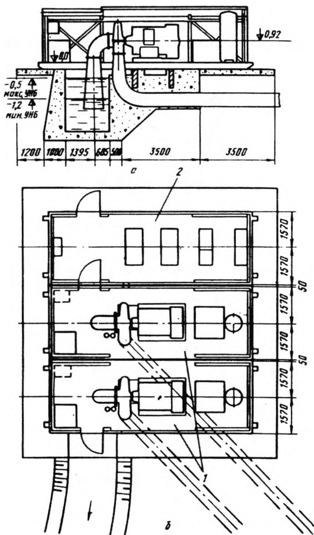
Рис. 5.19. Компоновка здания малой ГЭС из блок-секций a - разрез; б - план; 1 - агрегатная блок-секция; 2 - секция управления и автоматики
