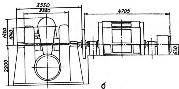
Рис. 2.8. Гидротурбины P075-B-140 (а) и P0180/872A-Г-65 (б)
