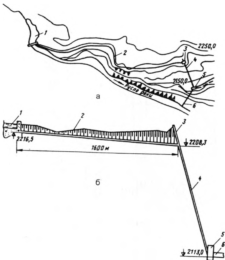
Рис.5.4. Компонка основных сооружений деривационной малой ГЭС
