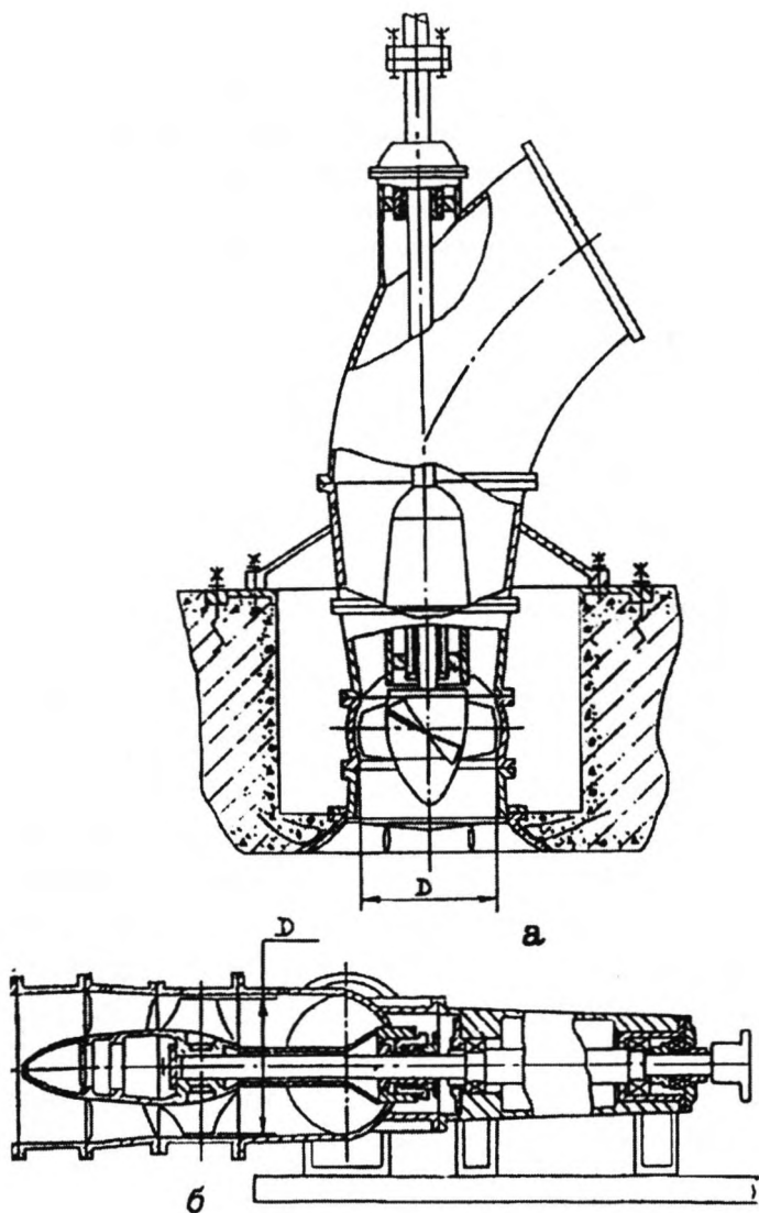
Рис.2.19. Вертикальные (а) и горизонтальные осевые (б) насосы, рекомендуемые для использования в обратимом режиме для МГЭС (завод "Уралгидромаш")
