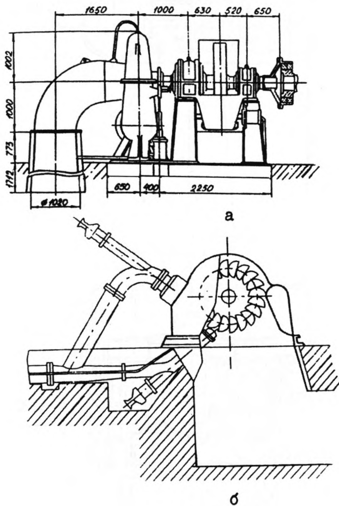
Рис. 2.10. Гидроагрегаты с гидротурбинами P0230/791Д-Г-71 (а) и КМ300Г-110 (б)
