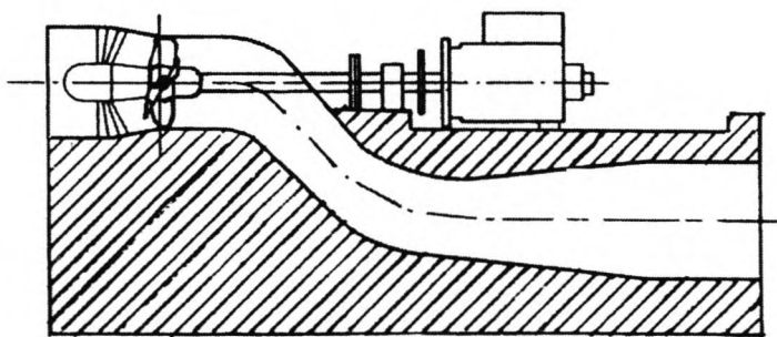
Рис. 2.11. Гидроагрегаты с гидротурбинами К400/685-Г2-114,3 (а) и ПЛ(ПР) М-820-160 (б)
