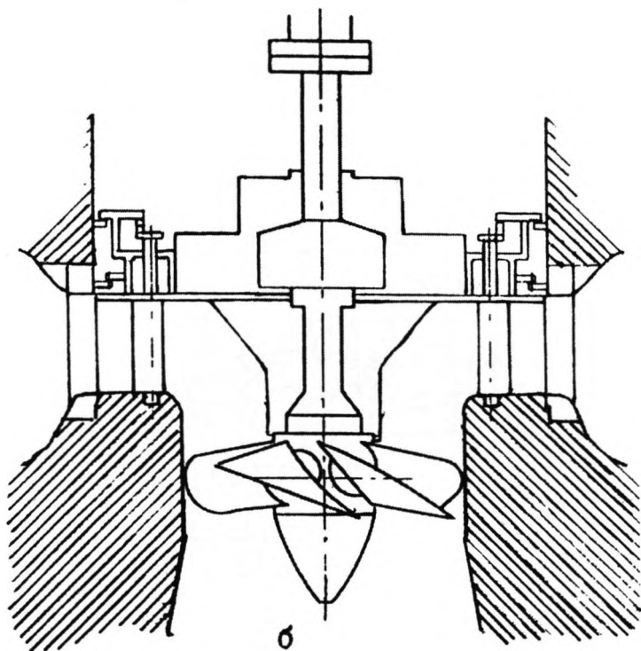
Рис. 2.5. Гидротурбины Р0180/872А-В-52 (а) и П Р30-В-160 (180)(б)
