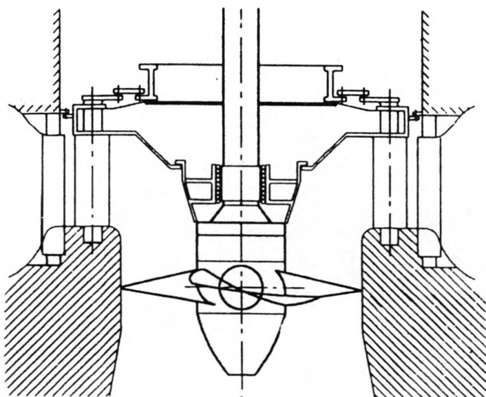
Рис. 2.3. Гидротурбины Р045/820-В-120 (а) и ПЛ120-В-280 (б)
