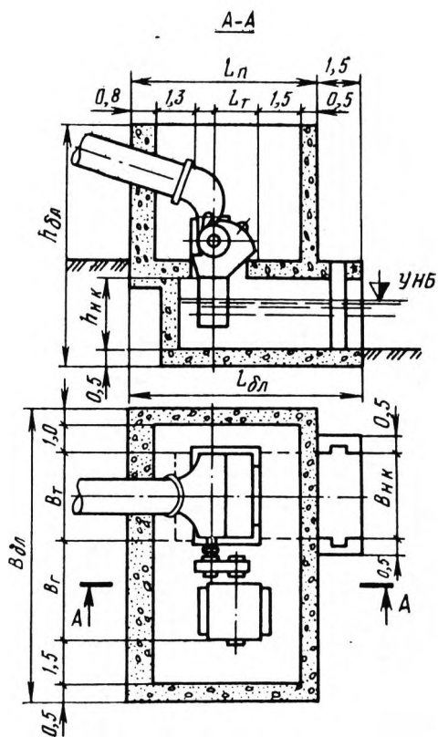
Рис. 5.13. Здание ГЭС с двукратной турбиной (типа Банки)
