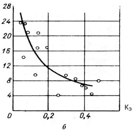
Рис. 1.1. Графики зависимости K_{\mathcal{E}}=f(\mathcal{E}/L)
