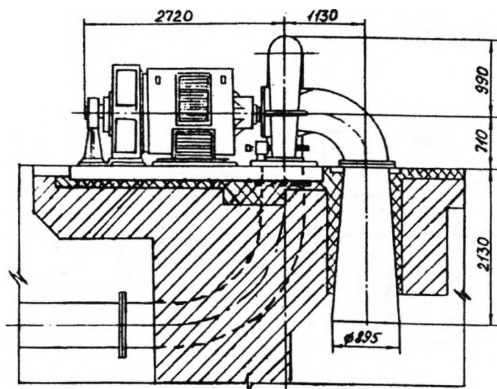
Рис. 2.7. Гидротурбина P075/728Б-В-160 (а) и гидроагрегат с гидротурбиной P023и/791Д-Г-50 (б)
