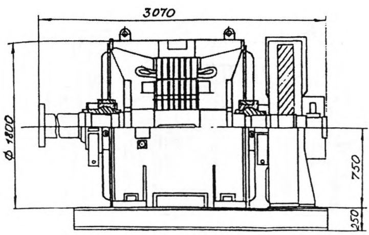
Рис. 2.18. Гидрогенераторы СГ143/72-14УХЛ4 (а) и СГ143/42-6УХЛ4 (б)
