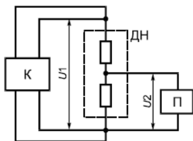
Схема измерения калибратором
