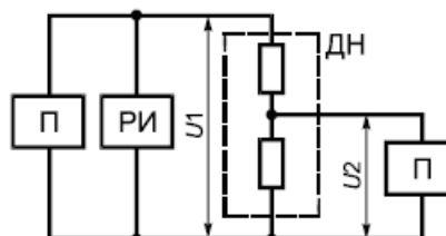
Схема измерения регулируемым источником постоянного напряжения
