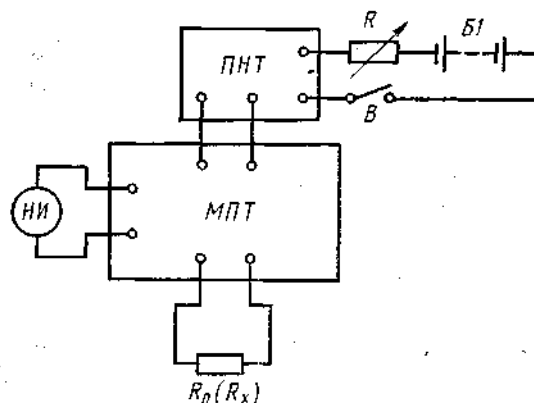
МПТ—мост постоянного тока; НИ—нулевой индикатор
