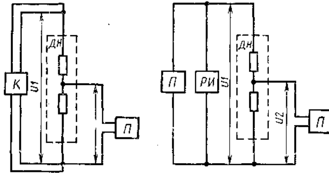
Схема измерения регулируемым источником постоянного напряжения
