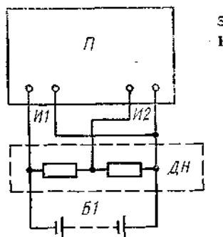
ДН—делитель напряжения Черт. 3
