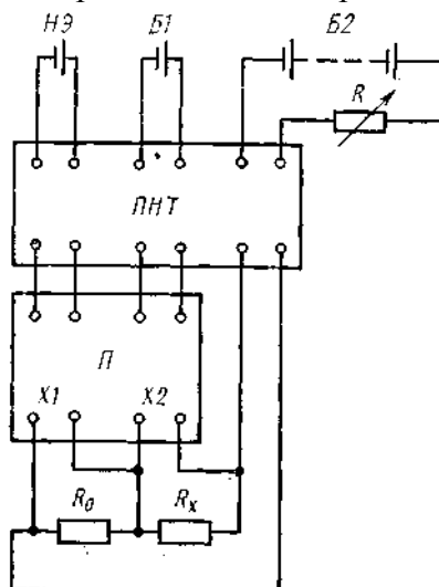
П —потенциометр постоянного тока; ПНТ —переключатель направления тока; R 0 —образцовая мера сопротивления; R x —измеряемое сопротивление; R —регулируемый магазин сопротивлений; HЭ —нормальный элемент; B1 , B2 —источники питания
