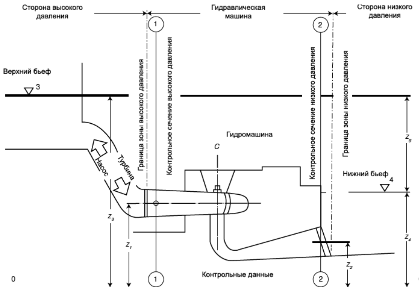
Рисунок 1 - Схема гидроэлектростанции
