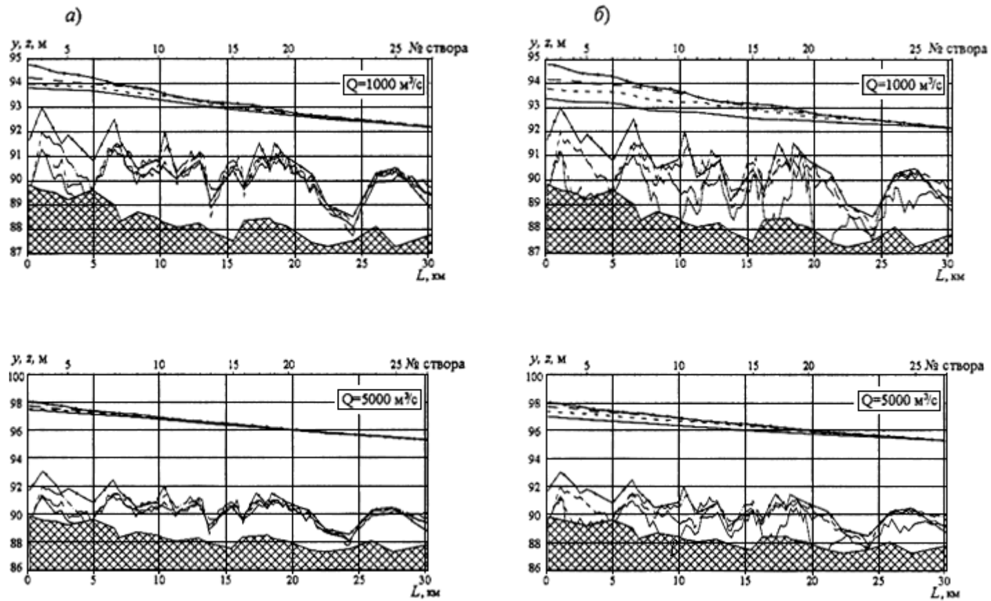
Рис.П4.5. Начальные и полученные расчетом уровни воды y(x) и продольные профили дна z(x) :
