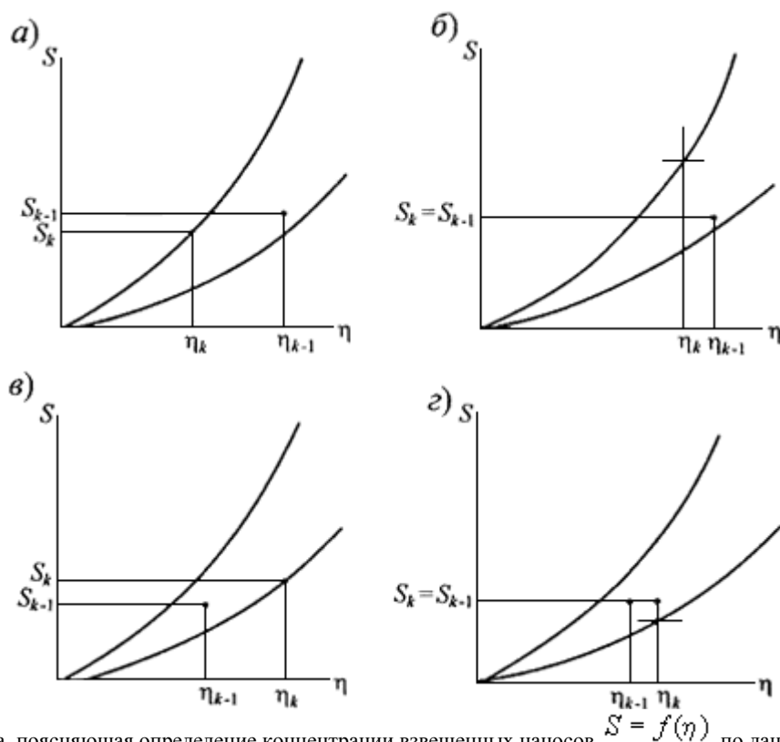
Рис.11. Схема, поясняющая определение концентрации взвешенных наносов S = f(\eta) по данным натуральных наблюдений
