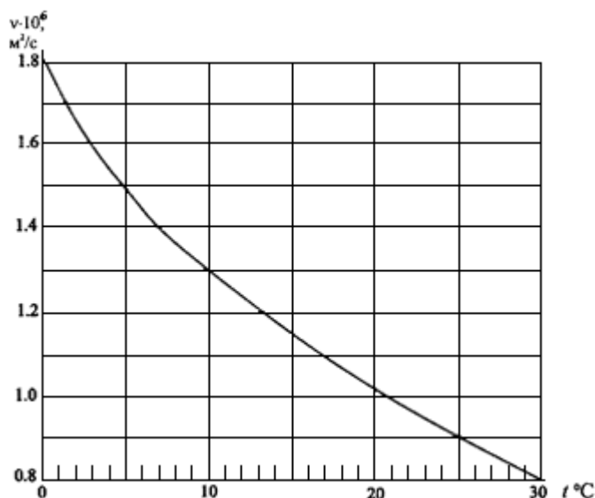
Рис.2. Зависимость кинематического коэффициента вязкости воды \nu от температуры t °C
