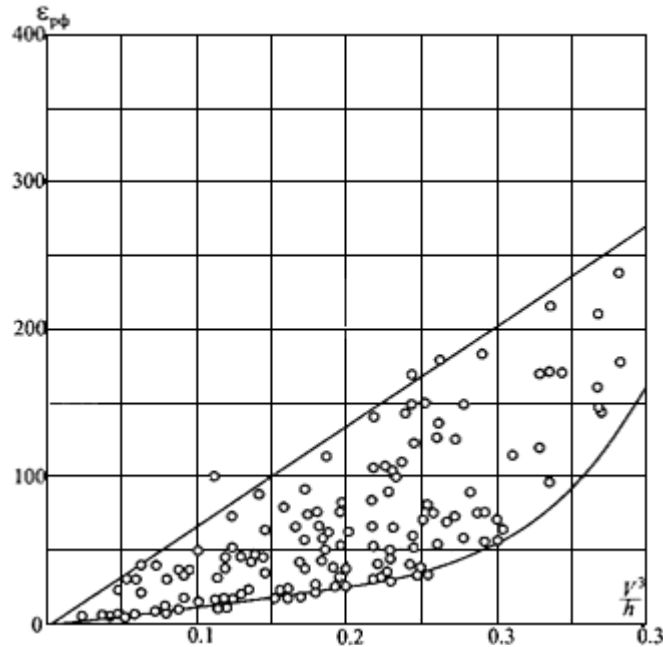
Рис.П2.1. Зависимость \varepsilon_{рф} = f(V^3/h)
