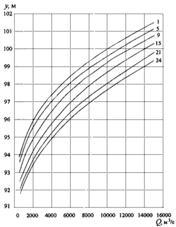
Рис.П4.1. Кривые связи расходов и уровней воды в опорных створах для примеров 1 и 2 в начальный момент:
