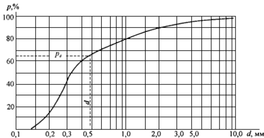
Рис.1. Кривая гранулометрического состава наносов
