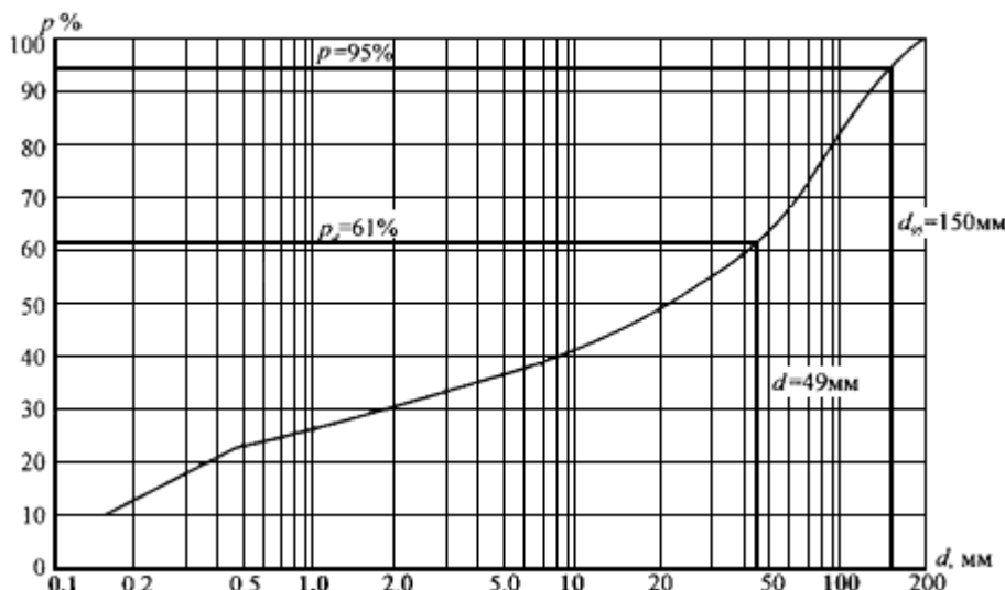
Рис.П3.1. Кривая гранулометрического состава наносов
