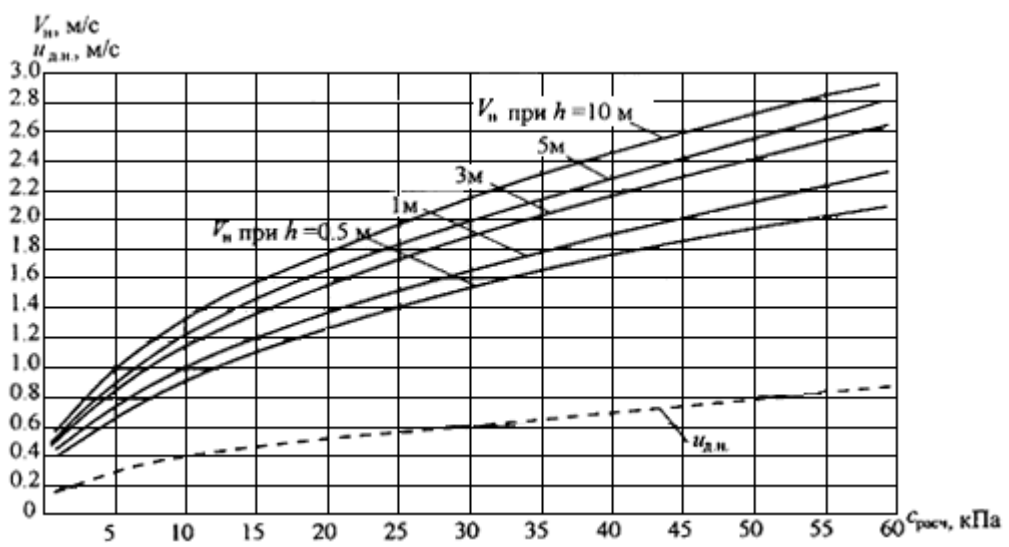
Рис.6. Зависимость неразмывающих скоростей V_n связных грунтов от расчетного значения сцепления
