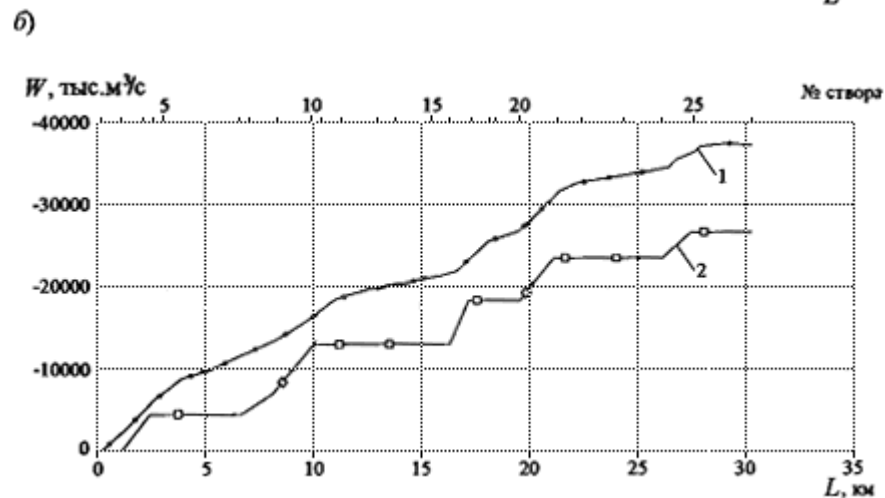
Рис.П4.6. Объемы деформаций (1) и карьерных разработок (2) русла за 1957-1976 гг.:
