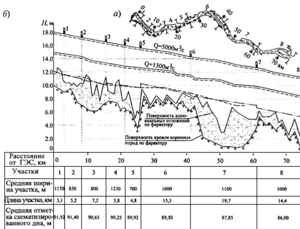
Рис.П1.1. Схематизация русла: план (а) и продольный профиль (б):
