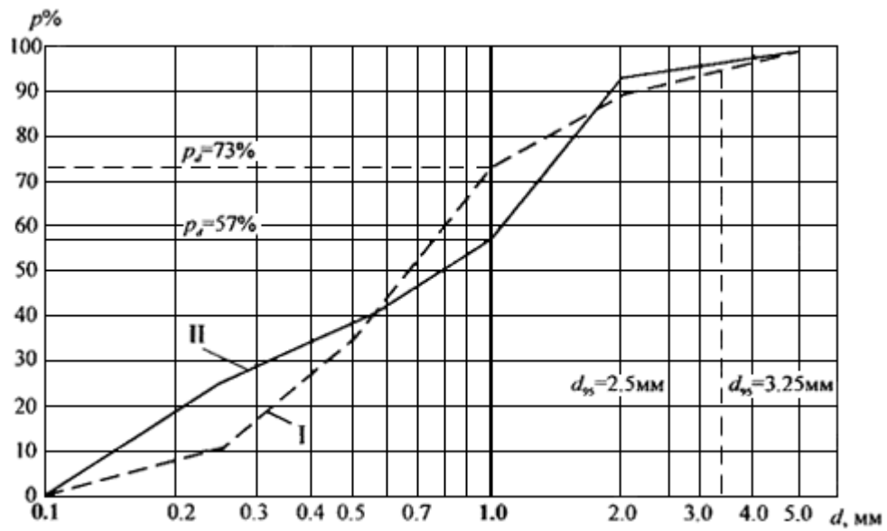
Рис.П5.1. Кривые гранулометрического состава разнозернистого грунта:
