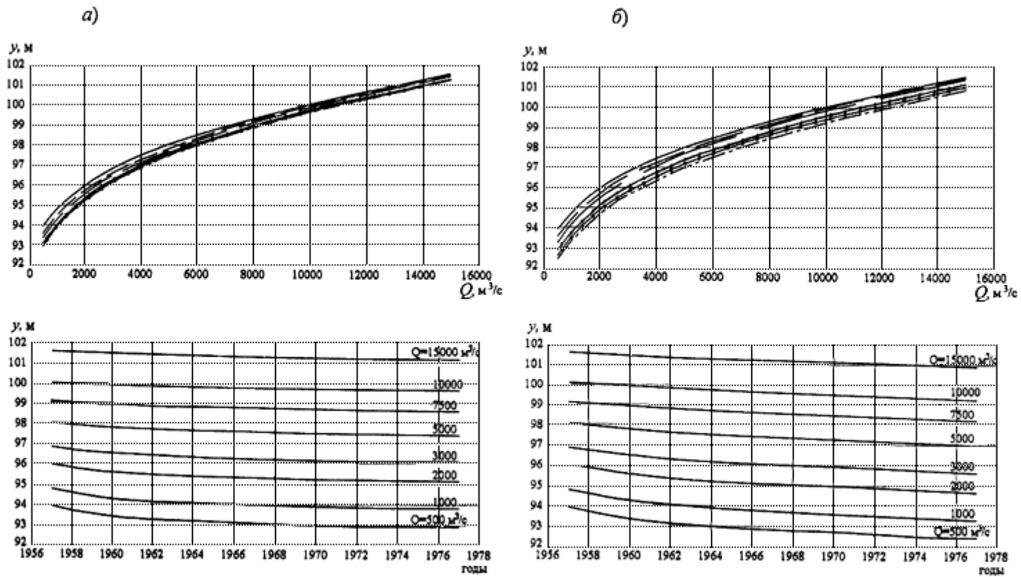
Рис.П4.2. Кривые связи расходов и уровней Q = f(y) и изменение уровней y в створе 1 при различных расходах Q :
