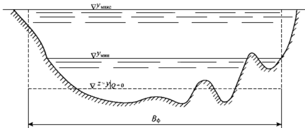
Рис.8. Схематизация живого сечения потока
