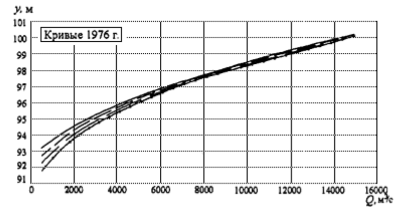
Рис.П4.4. Кривые связи расходов и уровней Q = f(y) и изменение уровней y в створе 15 при различных расходах притока Q_{\text{п}} на участке 18:
