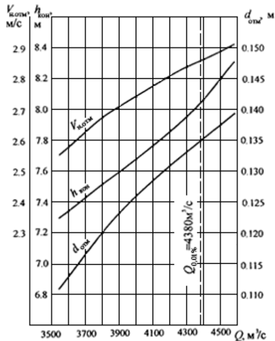
Рис.П3.2. Графики для нахождения параметров самоотмокания русла
