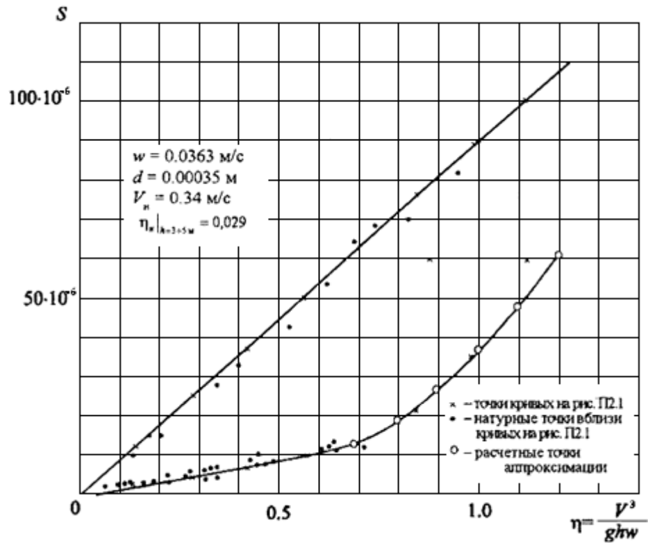
Рис.П2.2. Зависимость S = f(\eta)
