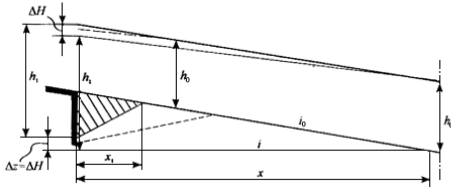
Рис.13. Схема расчета общего размыва по приближенному методу
