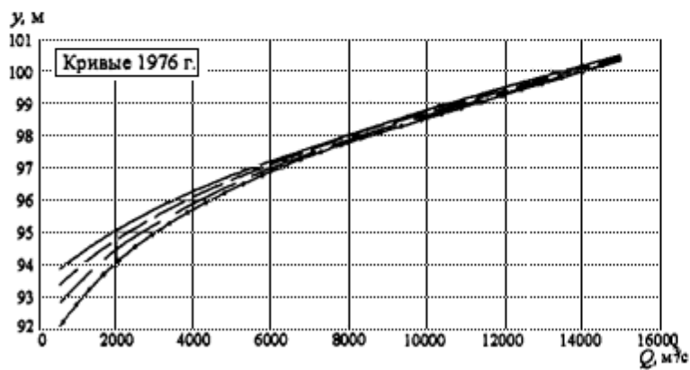
Рис.П4.4. Кривые связи расходов и уровней Q = f(y) и изменение уровней y в створе 15 при различных расходах притока Q_{\text{п}} на участке 18:
