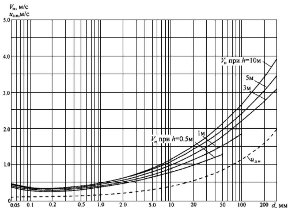
Рис.4. Зависимость неразмывающей скорости V_n несвязных грунтов от диаметра частиц d и глубины потока h (при
